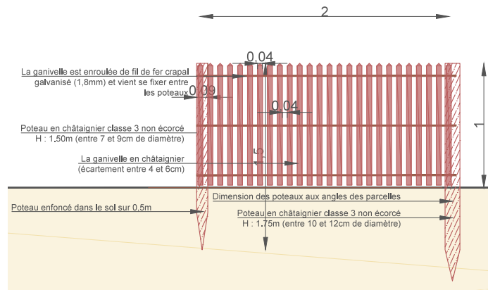
Clôture sur-mesure pour les jardins familiaux
