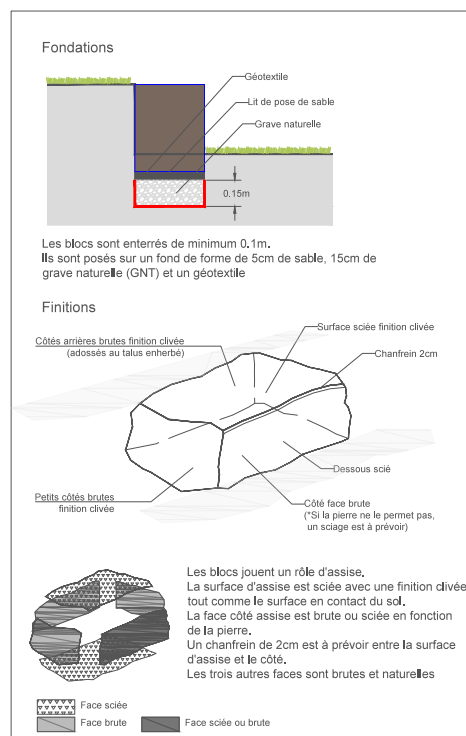
Dessin technique des gradins et dalles en granit
